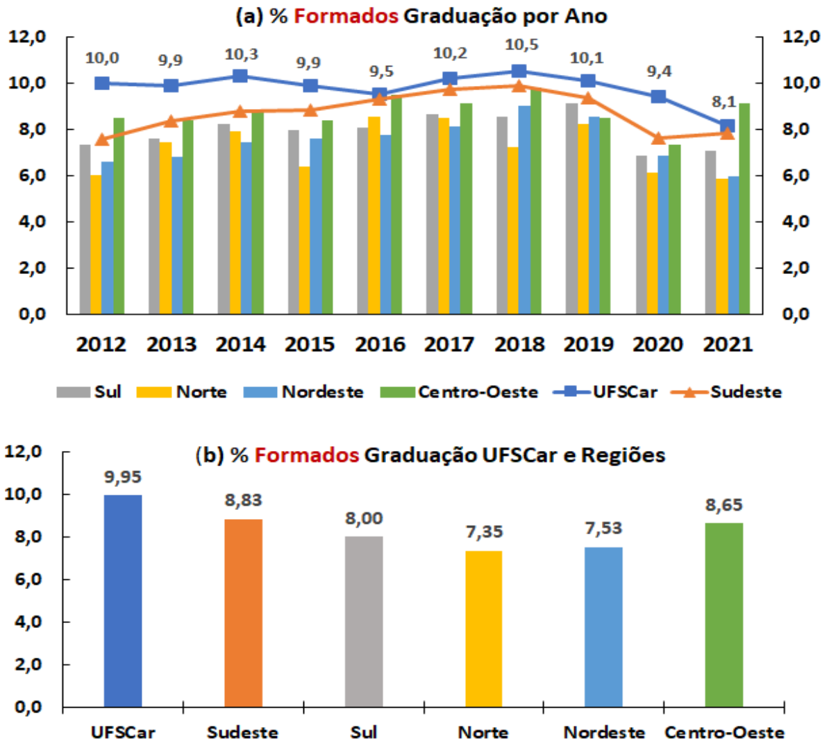
Figura 4 - Porcentagem de formados em cursos de graduação presencial, no período de 2012 a 2021. Na porção superior (a) temos a porcentagem de formados na UFSCar (linha), a mediana da porcentagem de formados da região sudeste (linha) e das demais regiões do País (colunas), para cada ano. Na porção inferior (b) temos a mediana da porcentagem de formados na UFSCar e das Universidades Federais das diversas regiões do País, nos 10 anos computados. (Fonte: Painel CoGrad/ANDIFES)
