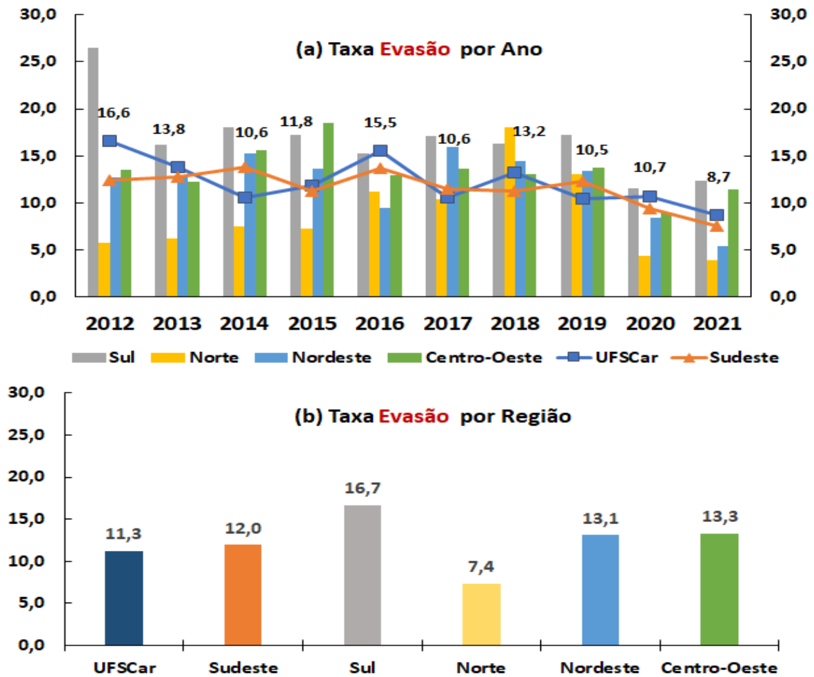
Figura 5 – Taxa de evasão UFSCar (linha), mediana da porcentagem de evasão da região sudeste (linha) e das demais regiões do País (colunas), no período de 2012 a 2021. (Dados coletados no Painel da CoGrad/ANDIFES)
